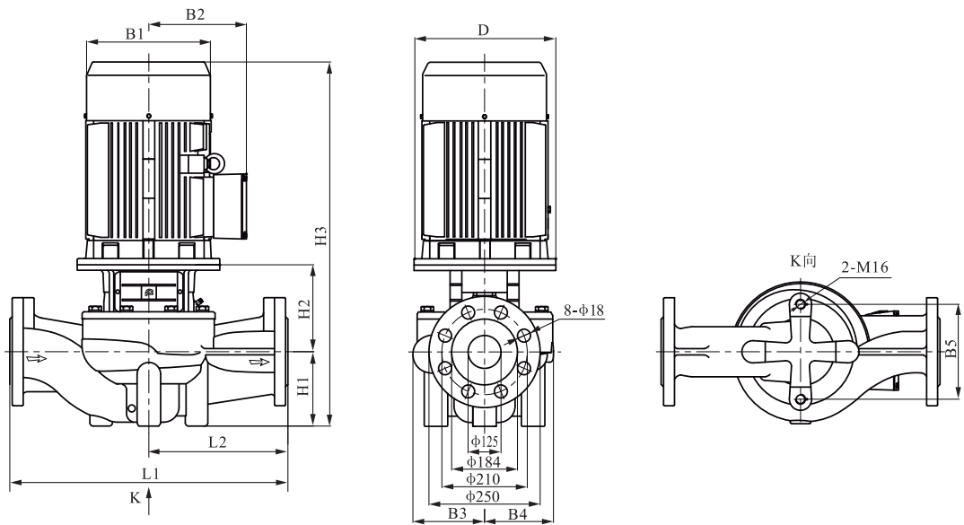
● Габаритно-присоединительные размеры и масса
